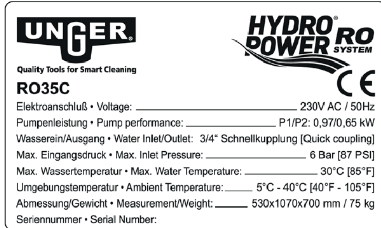
Abb. 1 Typenschild
