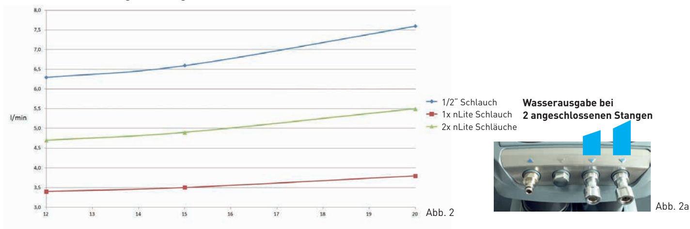
Abb. 2 Abhängigkeit der Leistung von Wassertemperatur und Schlauchdurchmesser bzw. Anzahl der Schläuche. Abb. 2a Bei zwei angeschlossenen Stangen erhält der rechte Wasseranschluß mehr Wasser von den Membranen als der Linke. Daher sollten längere Schläuche oder höhere Stangen rechts angeschlossen werden.
